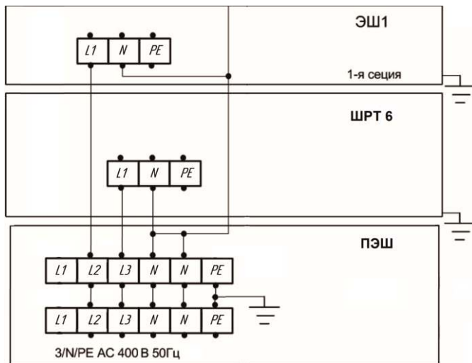
Рис. 9 Схема подключения шкафов ШРТ 4-ЭШ и ШРТ 6-ЭШ к модулям ЭШ-1
