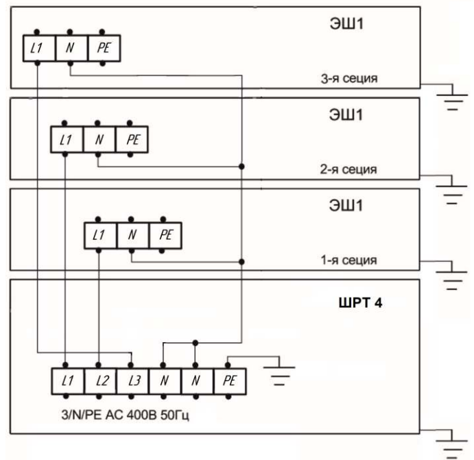
Рис. 9 Схема подключения шкафов ШРТ 4-ЭШ и ШРТ 6-ЭШ к модулям ЭШ-1
