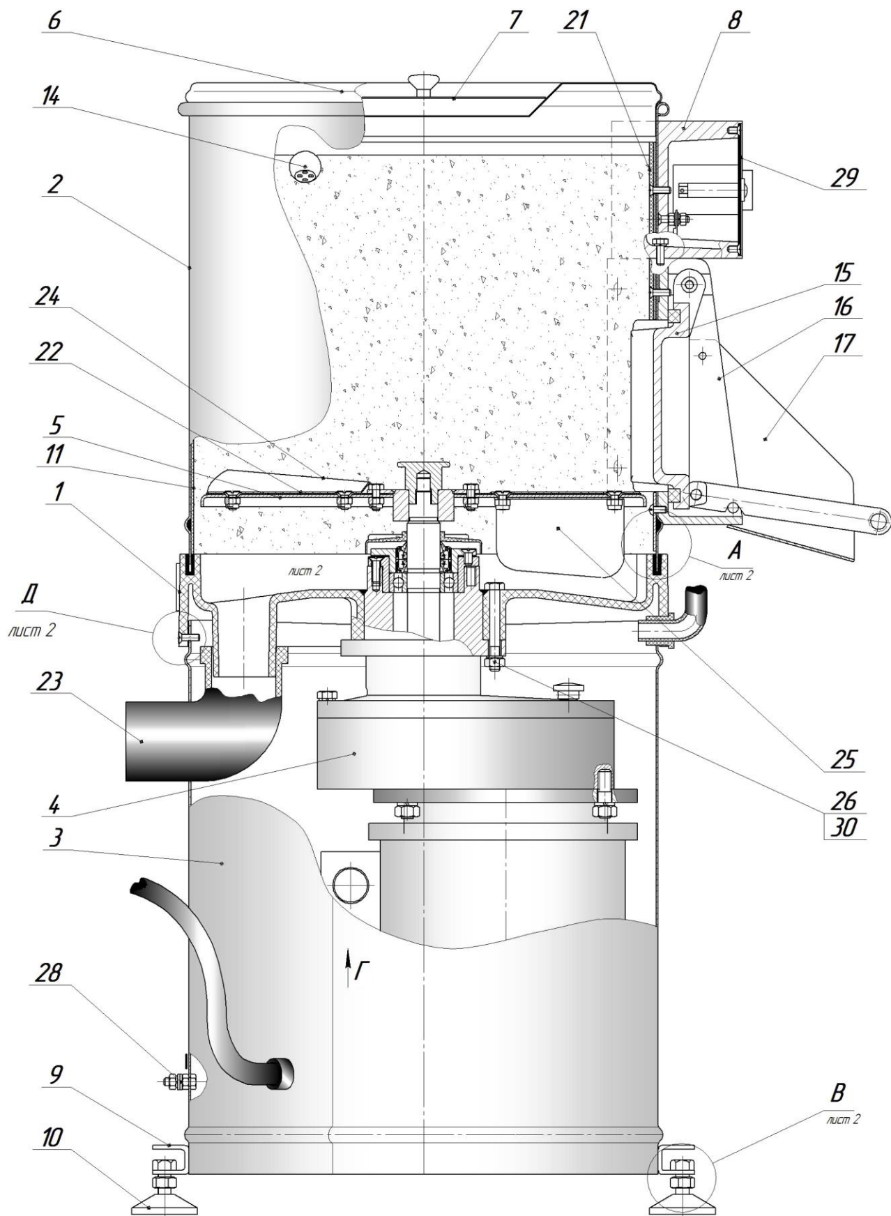
Рисунок – 1 Машина картофелеочистительная К-300 (лист 1)
