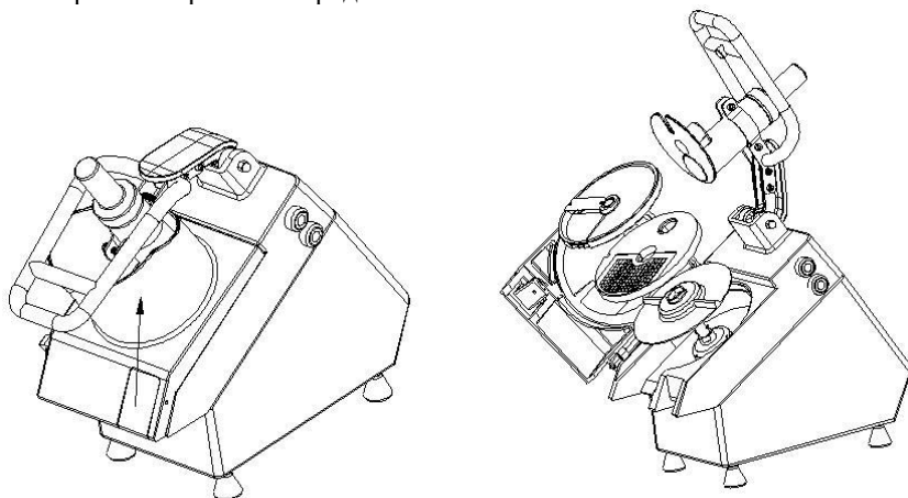
Рис.8 – Смена ножей
