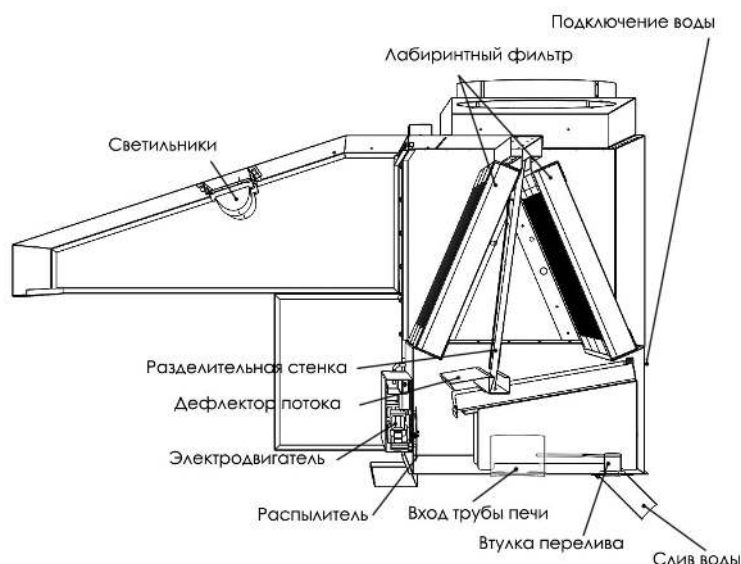
Рисунок 1. Гидрофильтр-искрогаситель
