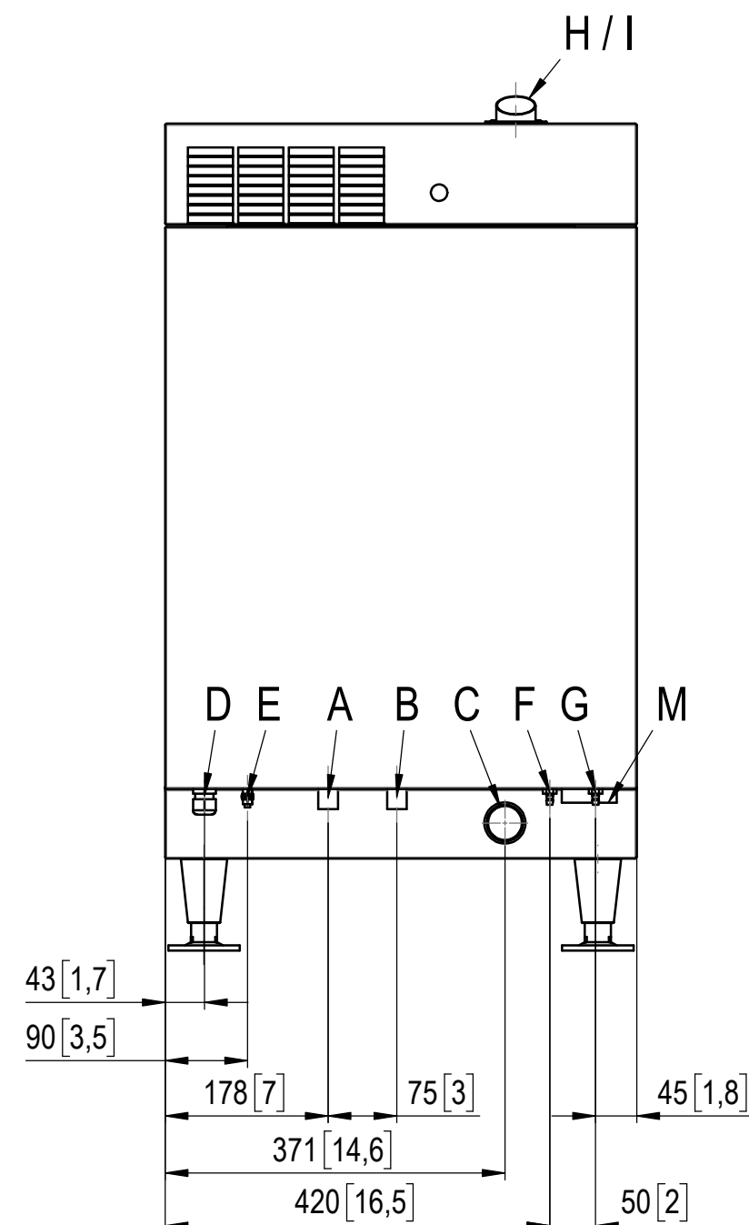
Ansicht von hinten / view from behind
