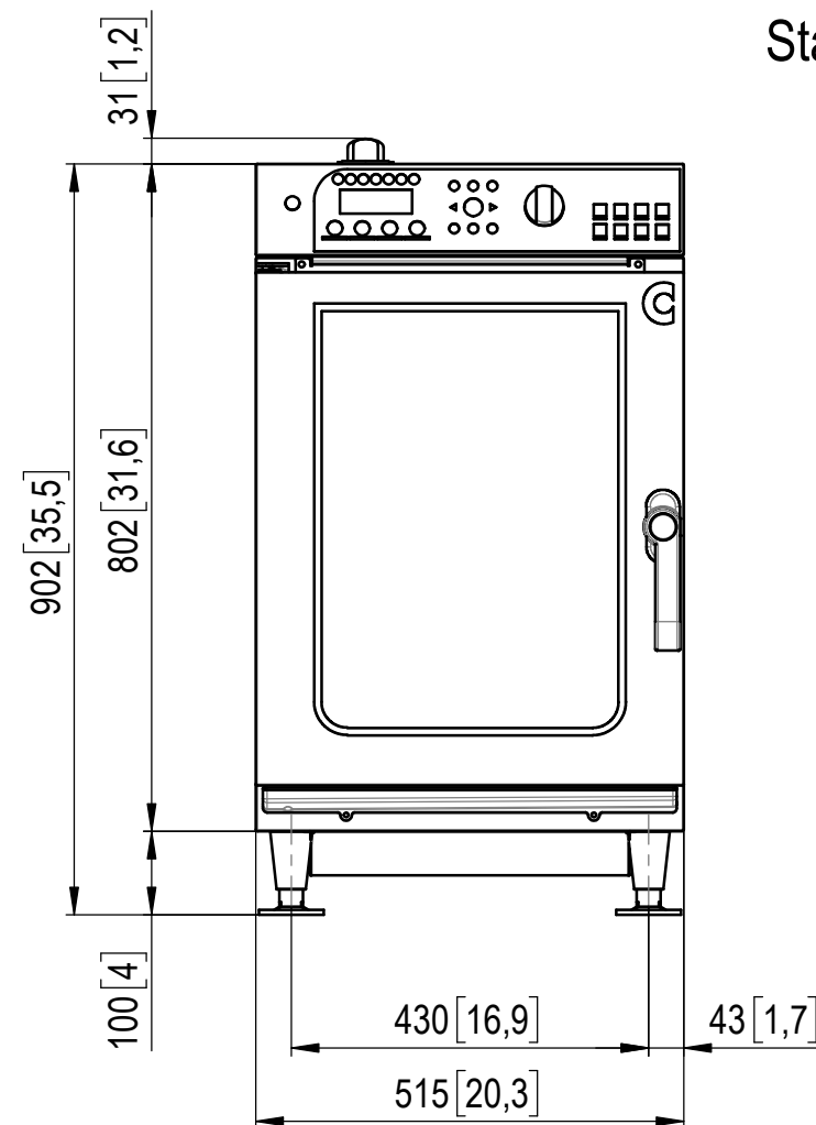
Vorderansicht Front view
