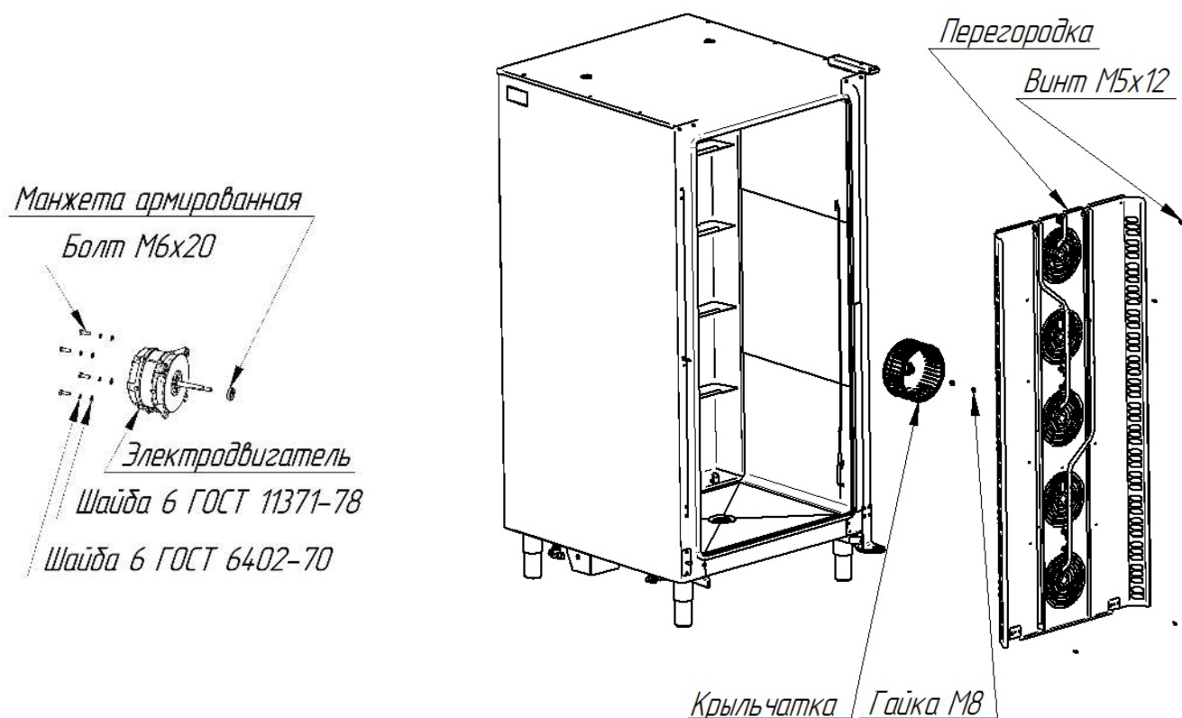
Рис. 11. Замена манжет
