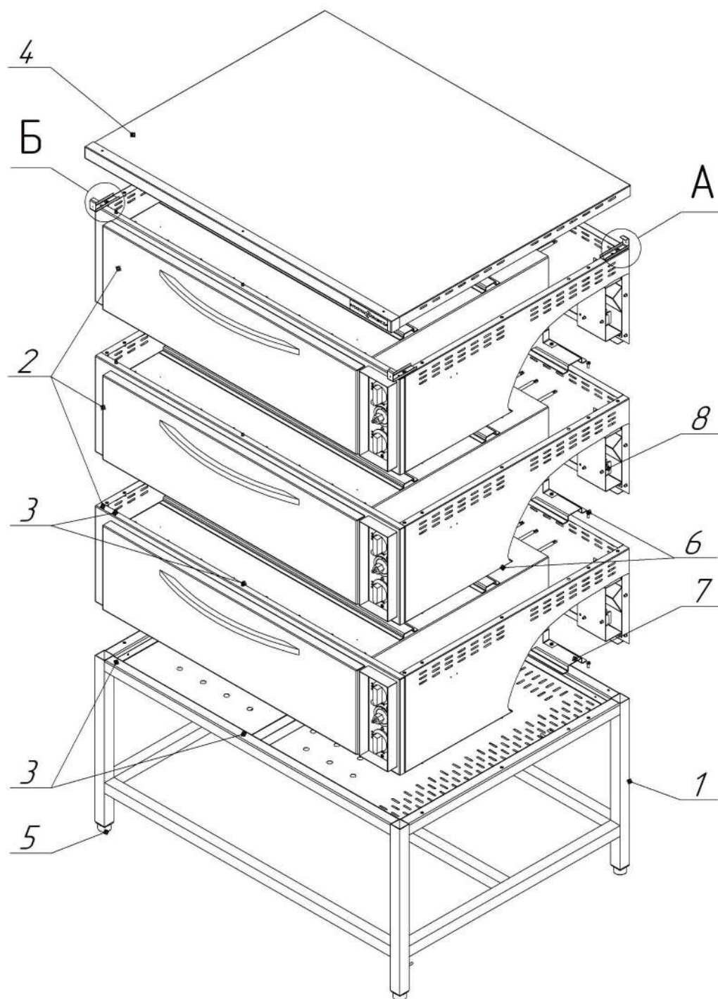
Рисунок 3. Схема сборки
