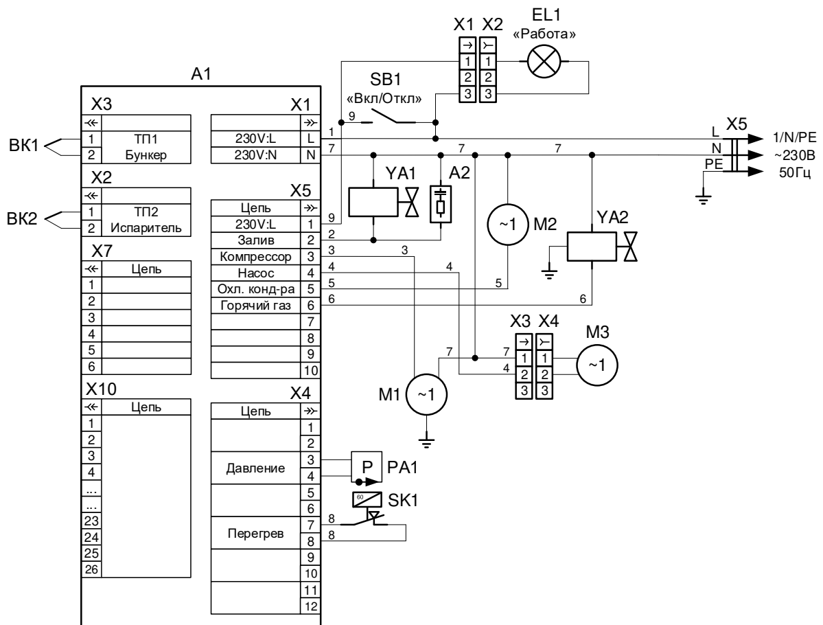
Схема электрическая соединений ЛГ-24/06К-02, ЛГ-24/06К-04 Допускается замена элементов, не ухудшающая технические характеристики изделия
