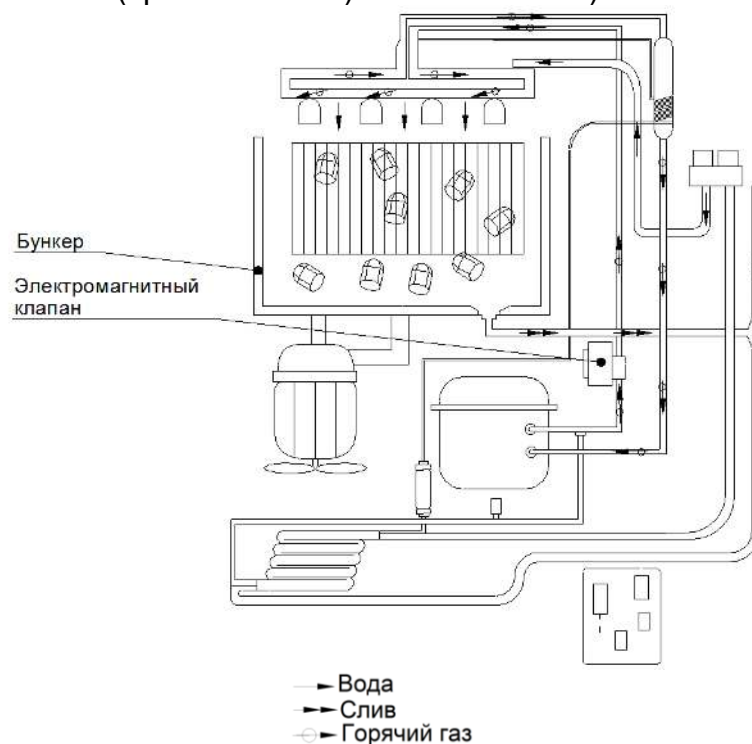
Рис. 3 Схема режимов работы льдогенераторов ЛГ-24/06К-01, ЛГ-24/06К-03
