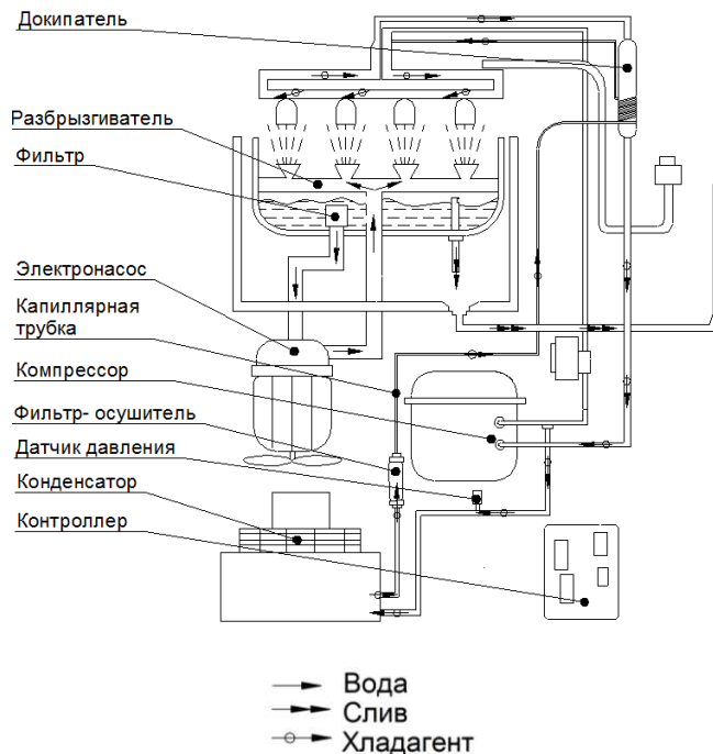
Рис. 3 Схема режимов работы льдогенераторов ЛГ-24/06К-01, ЛГ-24/06К-03
