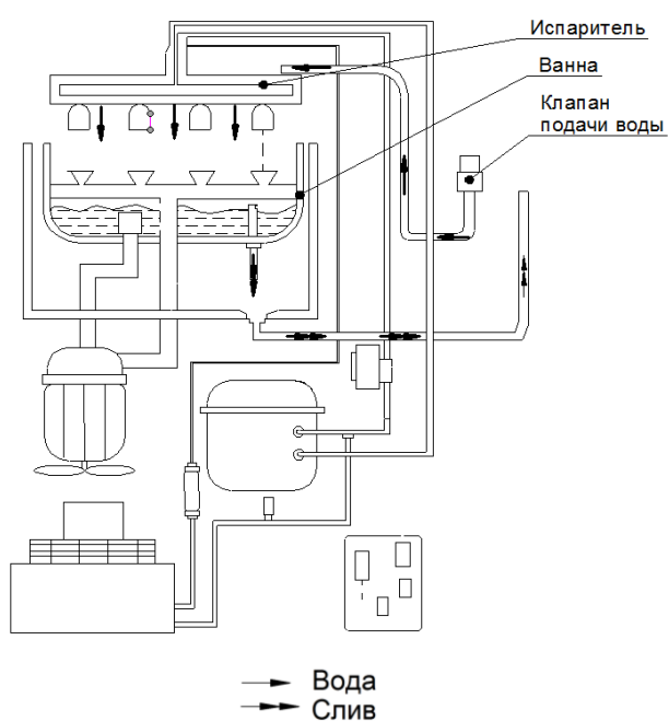
Рис. 3 Схема режимов работы льдогенераторов ЛГ-24/06К-01, ЛГ-24/06К-03
