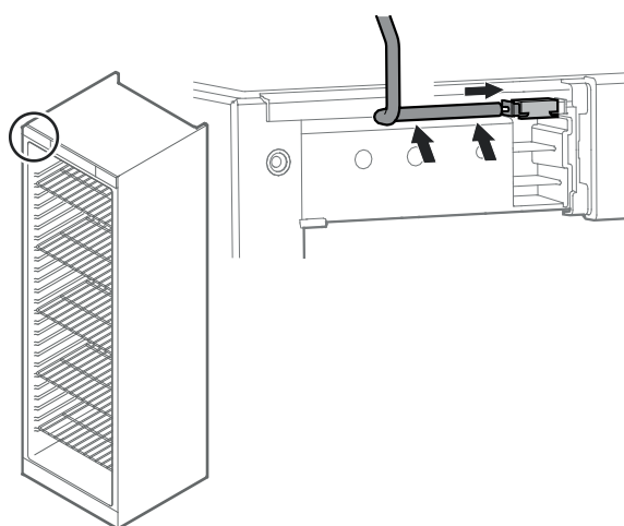
26. Вставьте штекер слева сверху.
