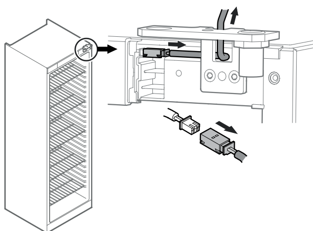
20. Вытащить штекер.
