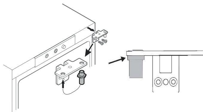
22. Открутить шарнирный уголок.
